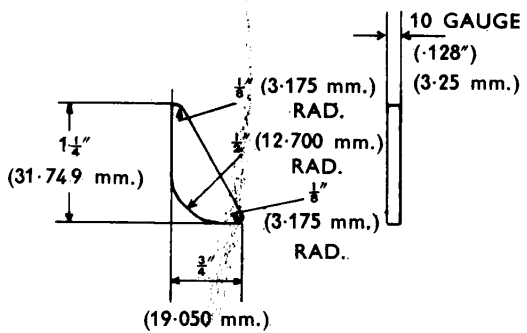
FIG. 3 STRAP STIFFENER B
